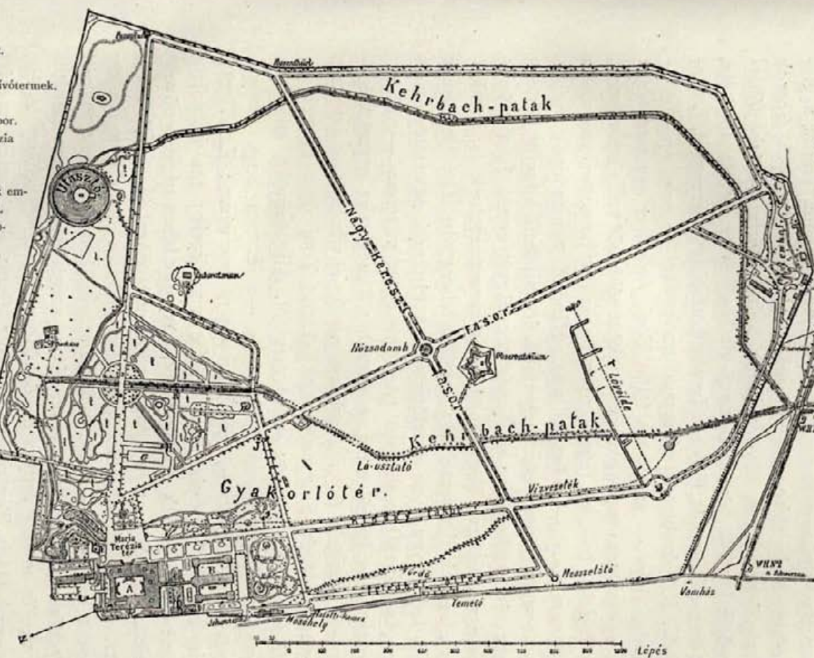
A bécsújhelyi katonaaikadémia tervrajza.
